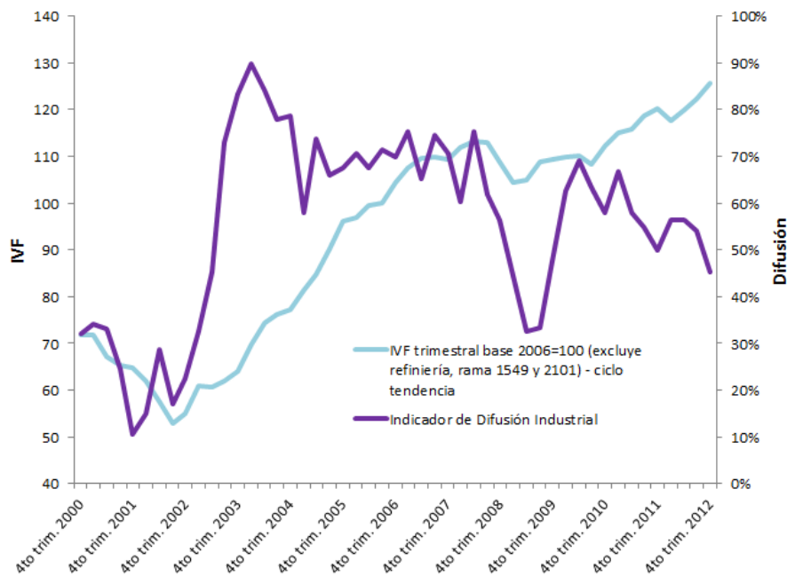
Gráfico 1.1 - Indicador de difusión de la producción industrial
