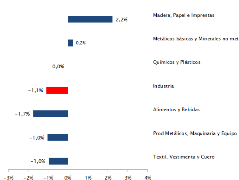
Gráfico 3 – Incidencia de la variación de la producción por agrupación industrial (4° trimestre 2012/2011)
