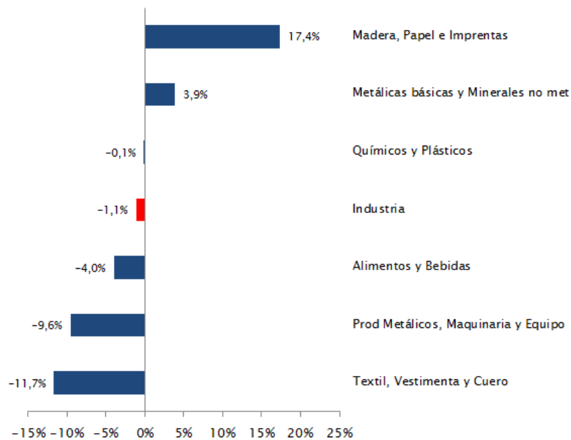
Gráfico 2 – Variación de la producción por agrupación industrial (4° trimestre 2012/2011)
